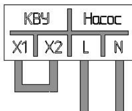
Рисунок 9 Схема подключения насоса и управляющего контакта
