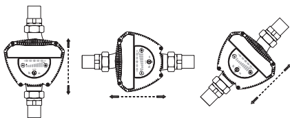
Рис. 4 Допустимое расположение вала насоса
