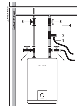
Рис. 5. Схема подключения к водопроводу моделей Genie ECO U
