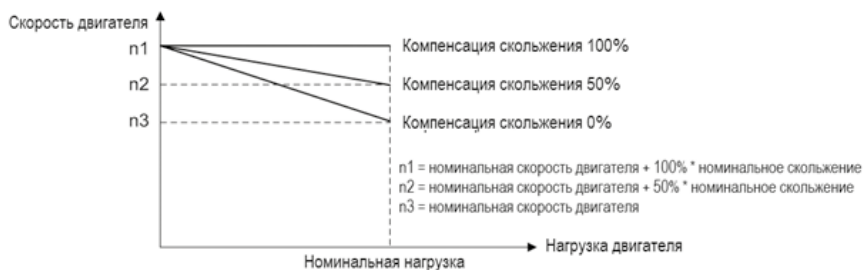
Компенсация скольжения в режиме вращения двигателя
