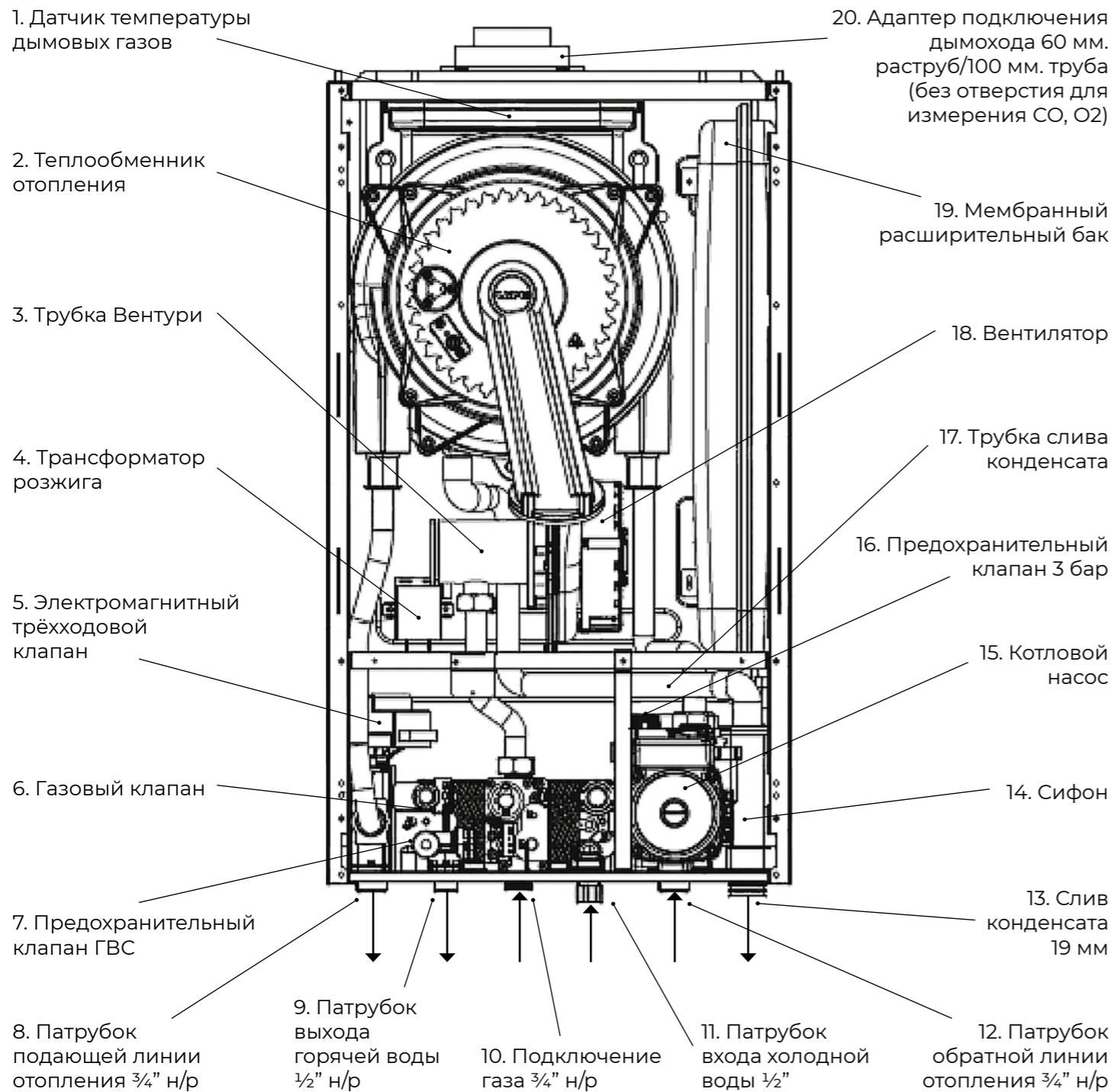
Рис. 2. Общая схема.
