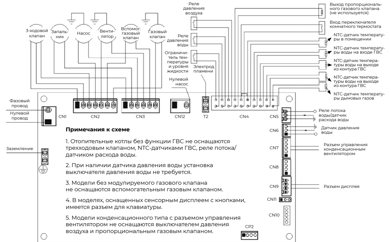
Рис. 26. Электрическая схема.
