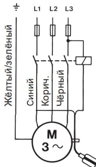
Трехфазное подключение
