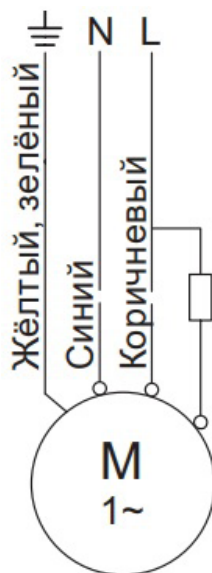
Однофазное подключение
