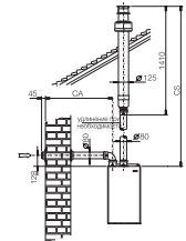
Раздельная система воздухозабора и вертикальным дымоотводом.
