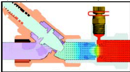
Фиксированная диафрагма
