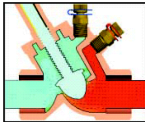
Переменная диафрагма
