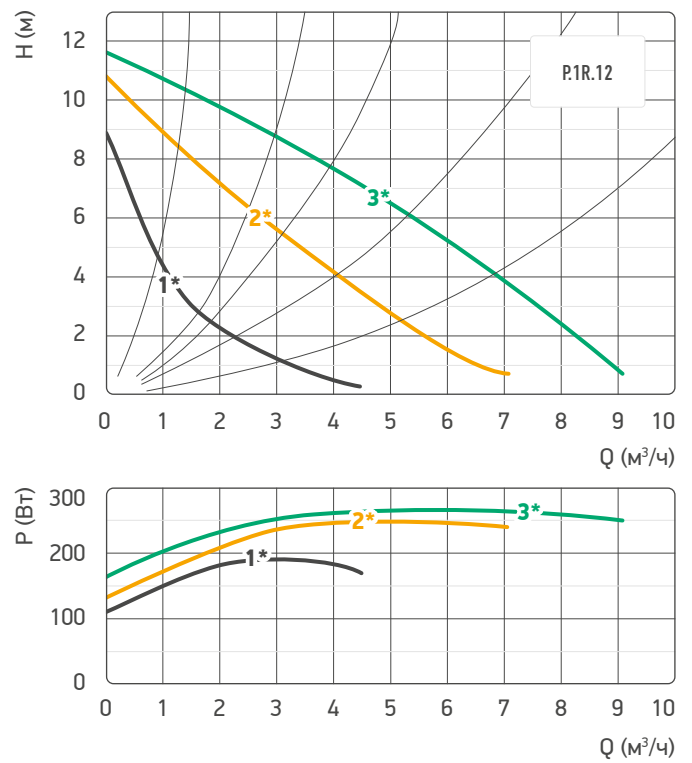
Гр. 4. Гидравлические характеристики насоса /P.1R.12
