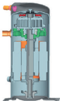
Спиральный компрессор
