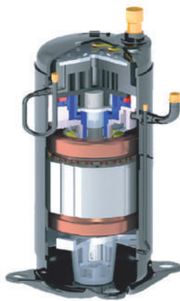
Герметичный спиральный компрессор
