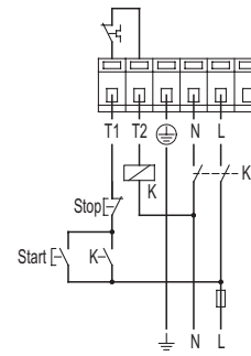
Рис. 18 Однофазный
