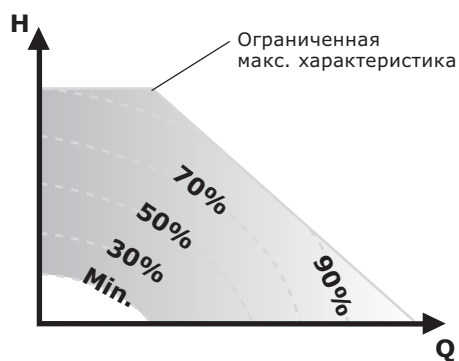
Рис. 54 Ограничения по мощности и давлению, влияющие на максимальную характеристику
