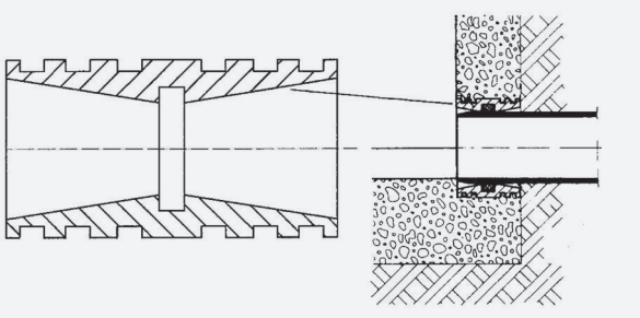
РИС. 13. ГИЛЬЗА ДЛЯ ПРОХОДА ЧЕРЕЗ СТЕНУ
