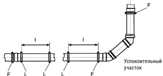
ПРИМЕРЫ РАСПОЛОЖЕНИЯ ЖЕСТКИХ И ПЛАВАЮЩИХ КРЕПЛЕНИЙ
