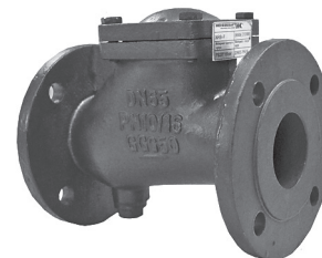
10 КЛАПАН ОБРАТНЫЙ ШАРОВЫЙ ФЛАНЦЕВЫЙ NRB-F
