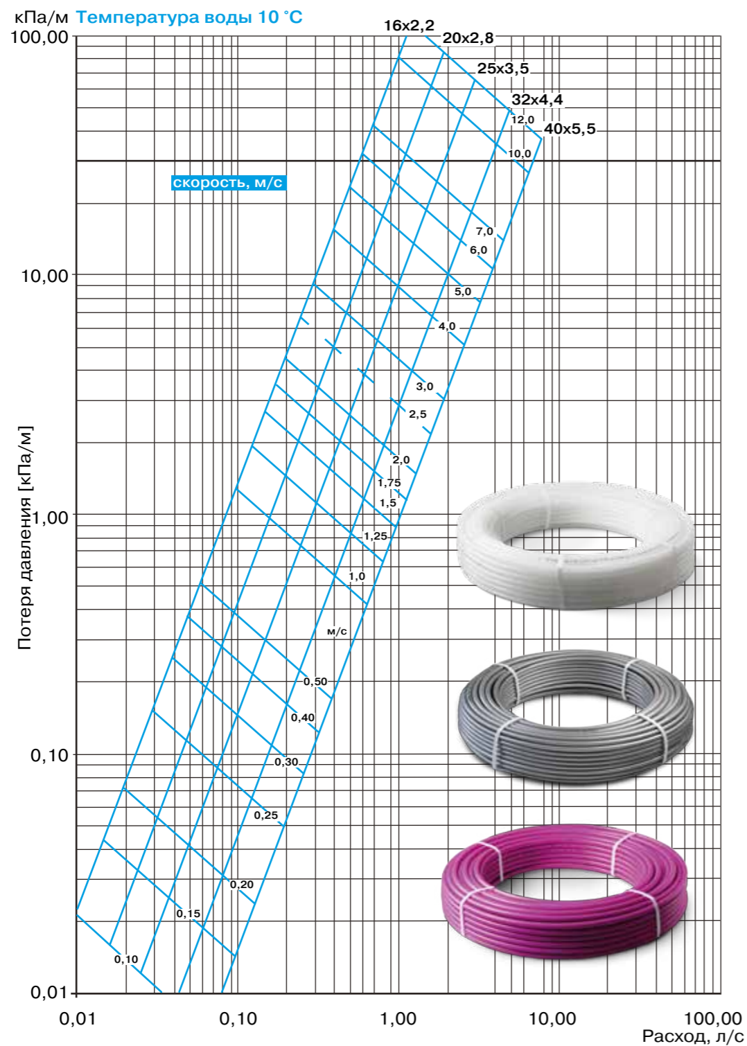
1. График линейных потерь давления в трубах PRO AQUA PE-Xa (серебристая) SDR 7.4 и PE-RT SDR 7.4 (белая)
