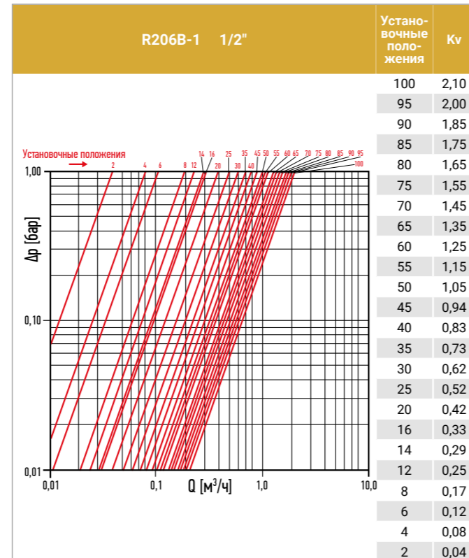
Диаграмма зависимости потерь давления от расхода по линии С-Д с отводом Ду 15 при установке ремонтной вставки
