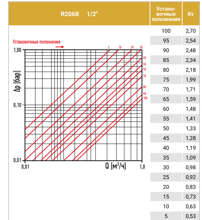
Диаграмма зависимости потерь давления от расхода для клапана партнера
