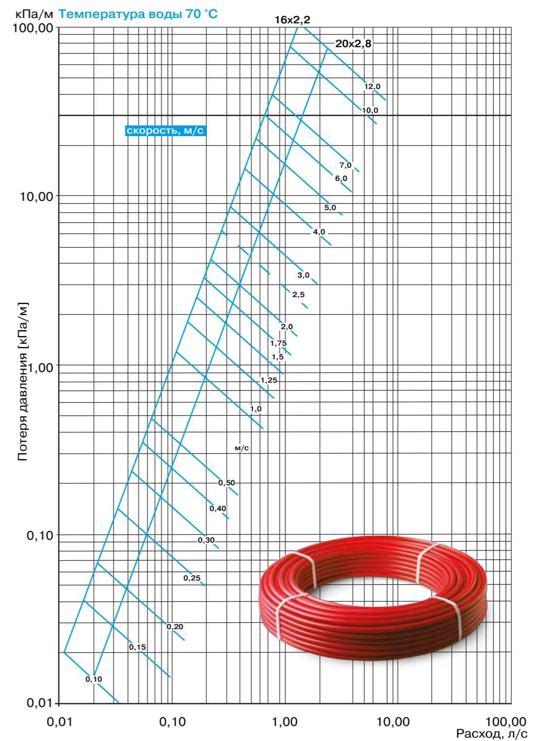
2. График линейных потерь давления в трубах PRO AQUA PE-Xa (красная), S3.5 / S4.5
