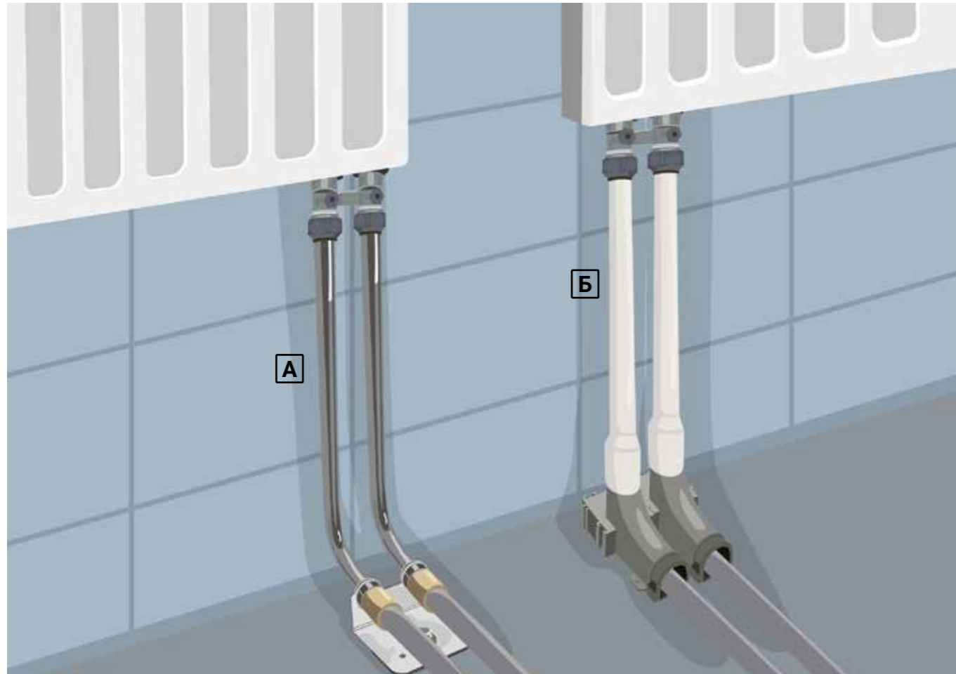
Способы подключения к радиатору с помощью: а - кронштейна для фиксации Г-образных трубок, б - фиксатора поворота трубы "башмак"
