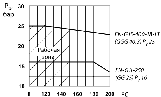
Зависимость рабочего давления от температуры перемещаемой среды
